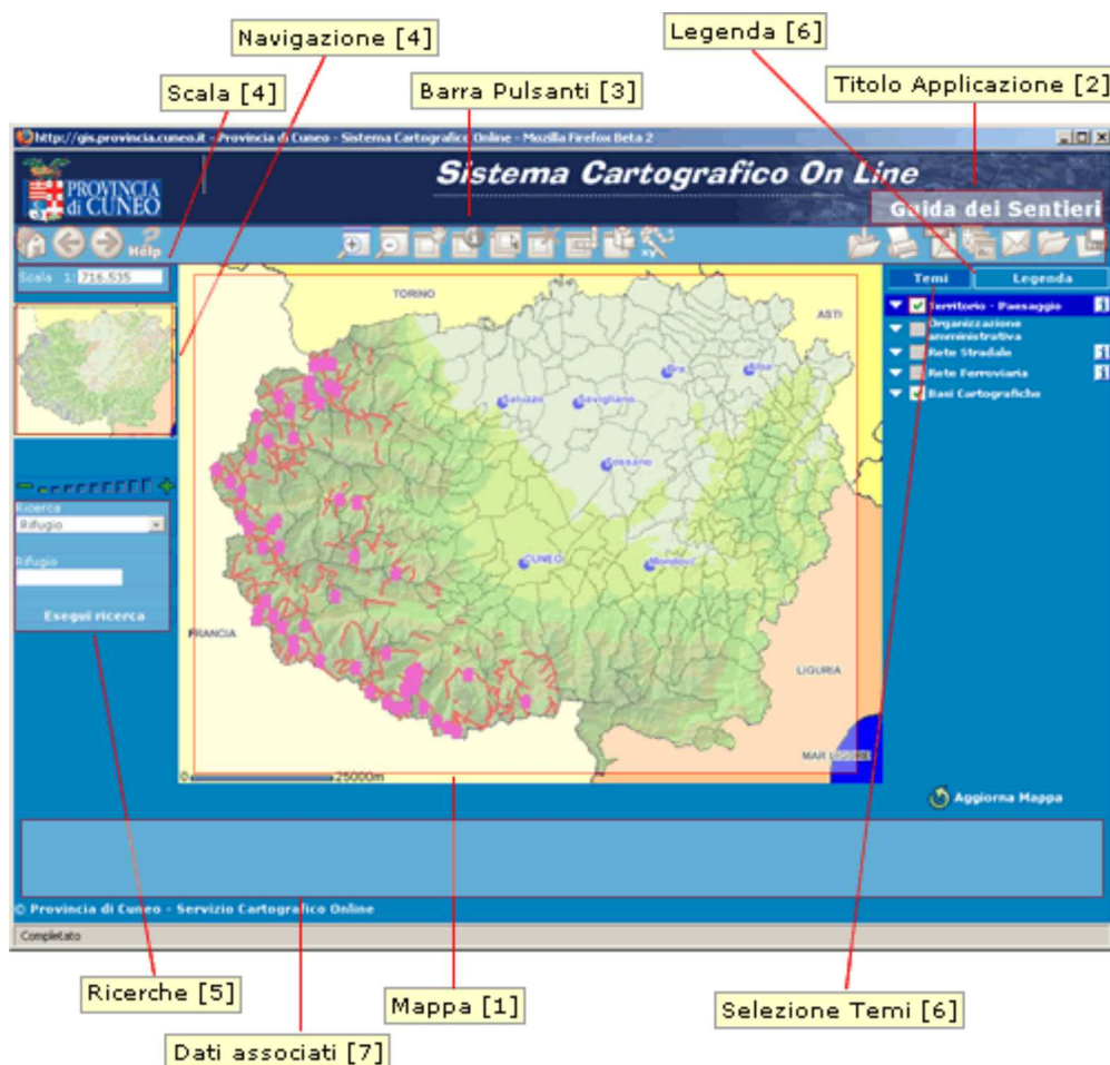
Figura 1 - Struttura dell'applicazione
